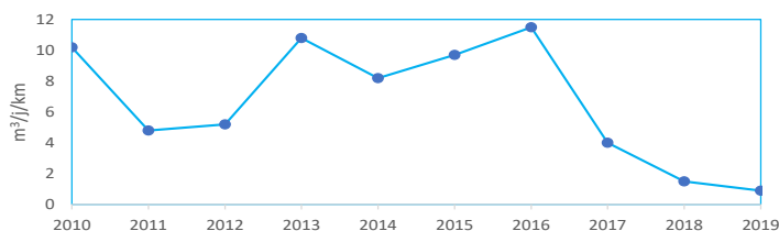
Evolution de l'indice linéaire des pertes en réseau
